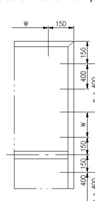
Ościeżnica okna z poprzeczką poziomą
