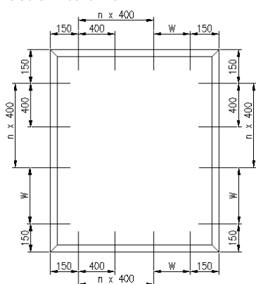
Ościeżnica okna
