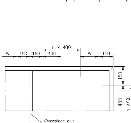
Ościeżnica okna z poprzeczką pionową
