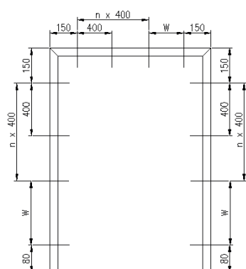
Ościeżnica drzwi
