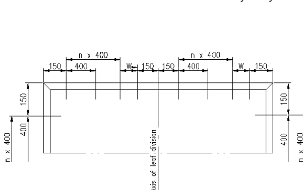
Ościeżnica drzwi 2-skrzydłowych
